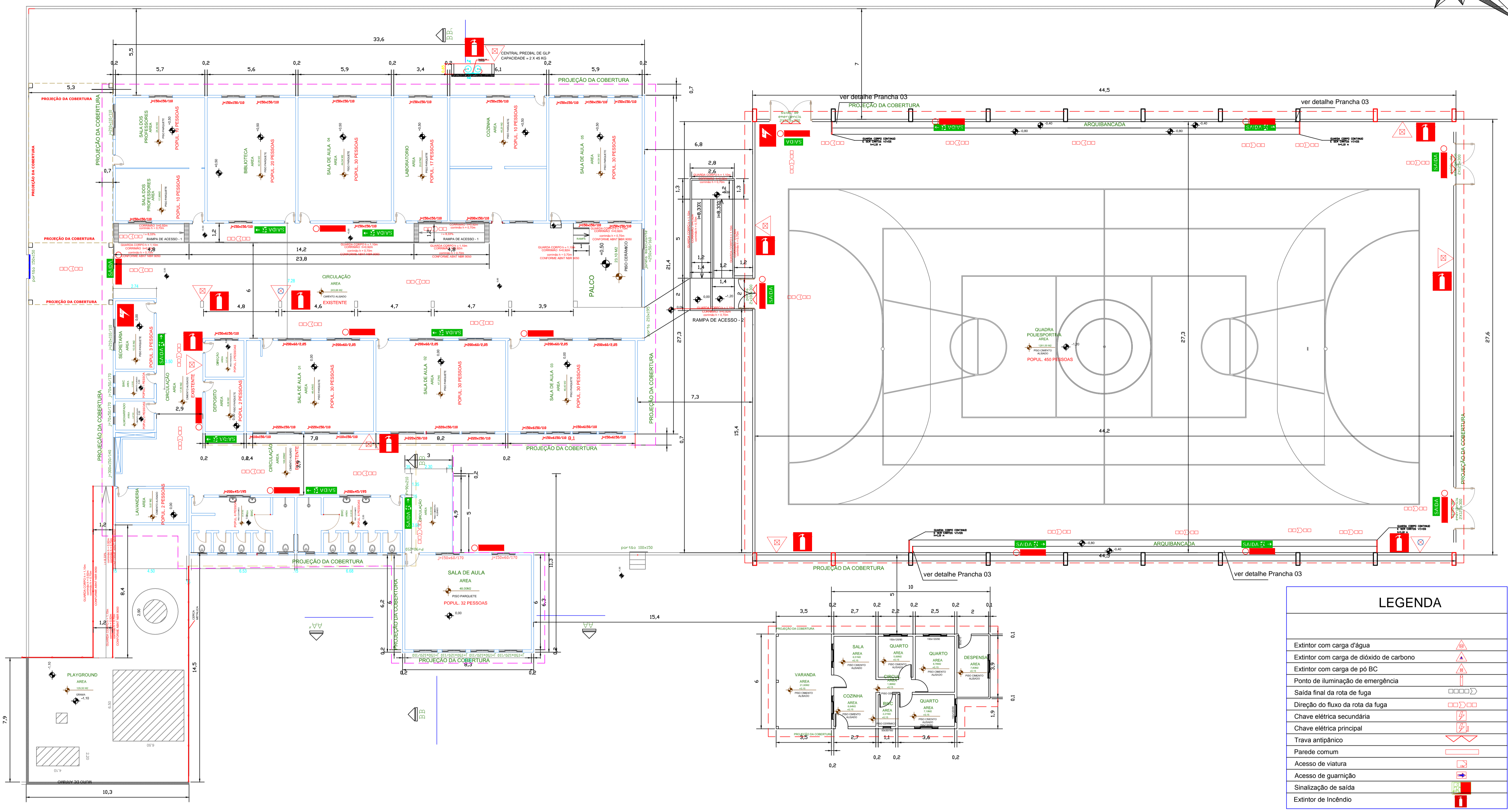
PLANTA BAIXA ESCALA 1: 125
